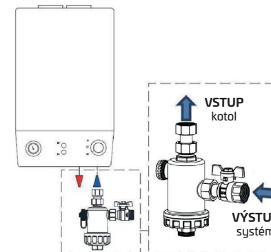
Schéma 2: Použitie magnetického filtra s hlavnou kazetou/telesom filtra smerujúcimi nadol
