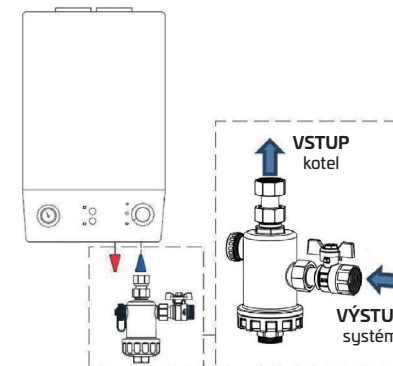
Schéma 2: Použití magnetického filtru s hlavní kazetou / tělesem filtru směřujícími dolů
